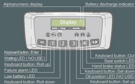
ZAPI Display
